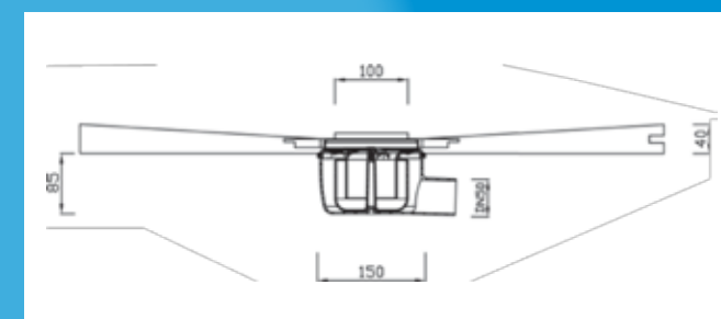
Basic Board met horizontale afvoer
