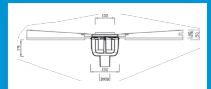
Basic Board met verticale afvoer
